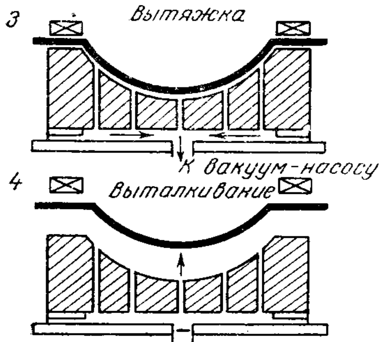
Рис. 8,8. Формование в матрице.
