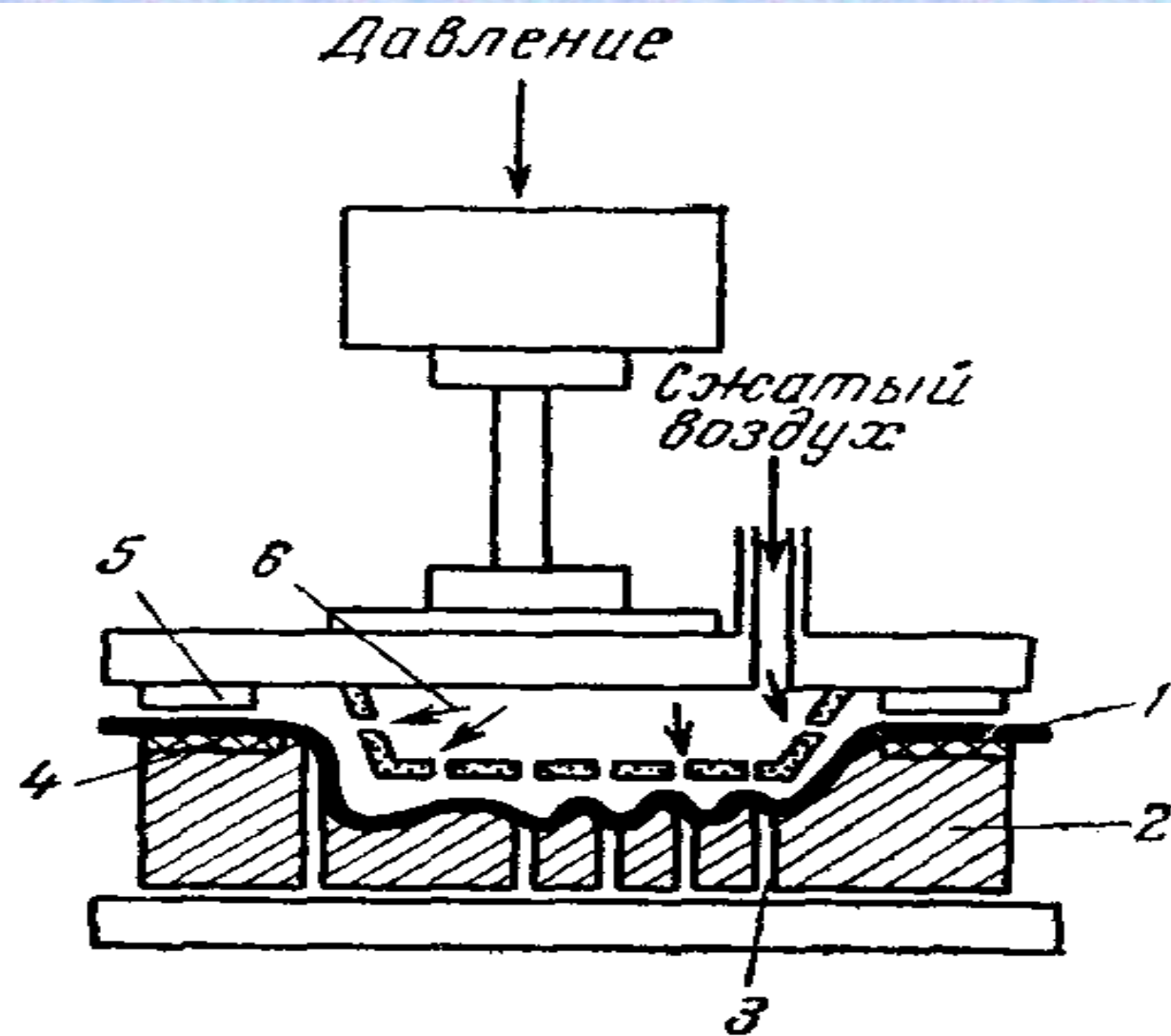
Рис. 8,4. Пневмоформование с применением толкателя:
